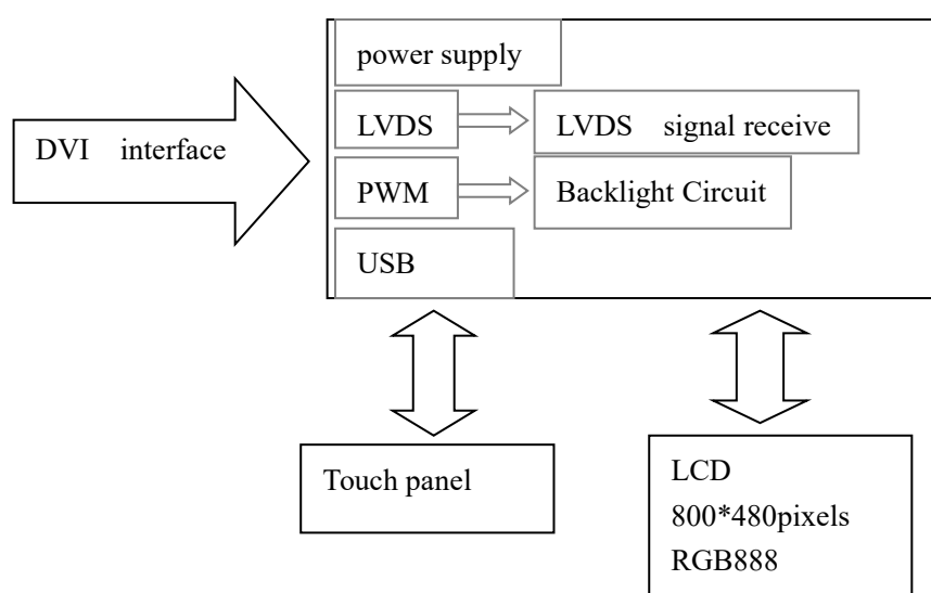
图 2.1.Block Diagram
