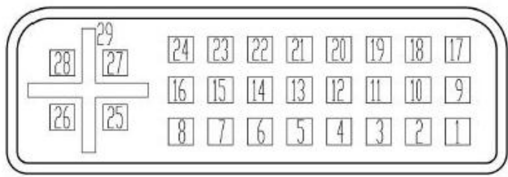
(图 1.1) 29PIN DVI-I 接口引脚定义 (P1)
