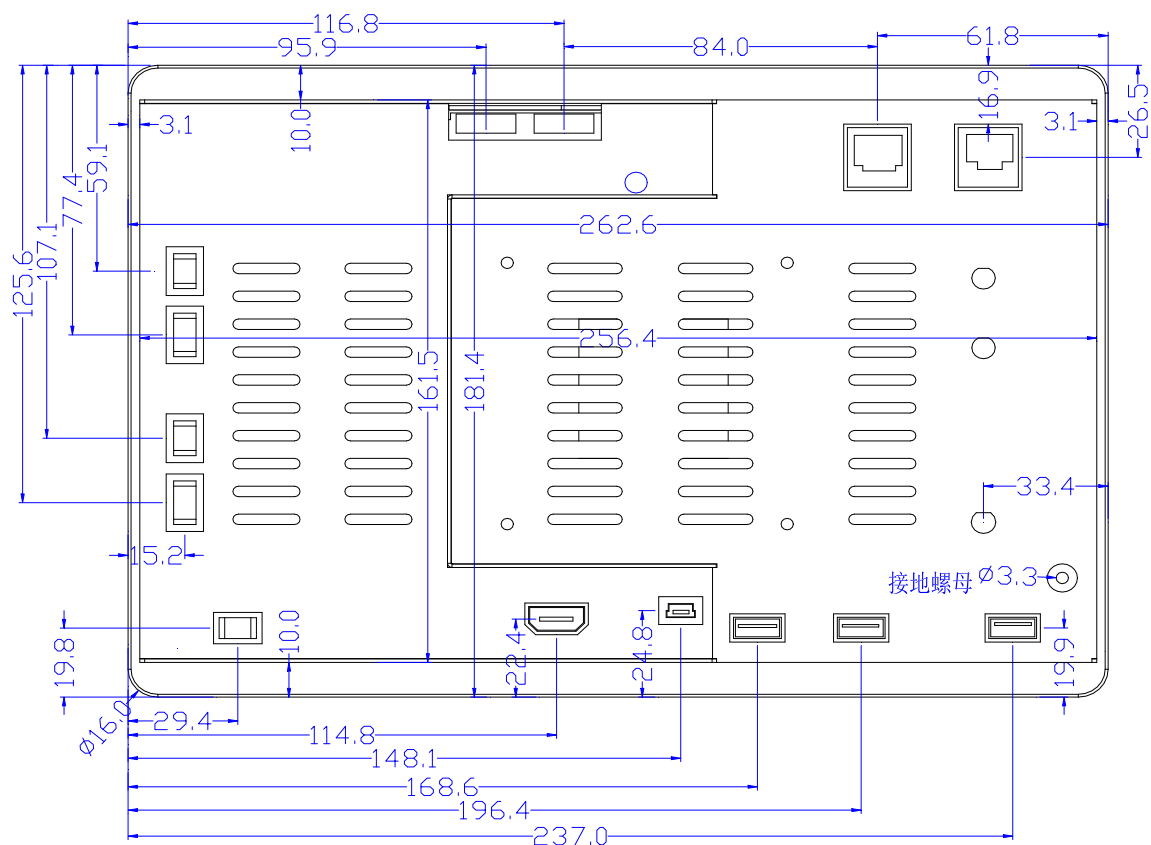
③背面整机示意图
