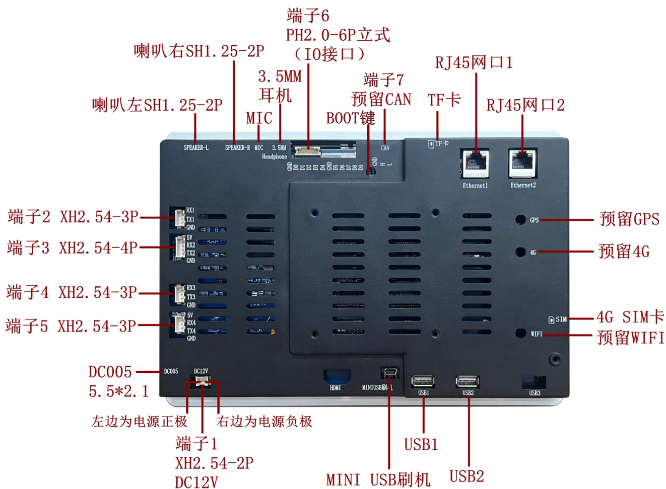
图-3 接口资源图解
