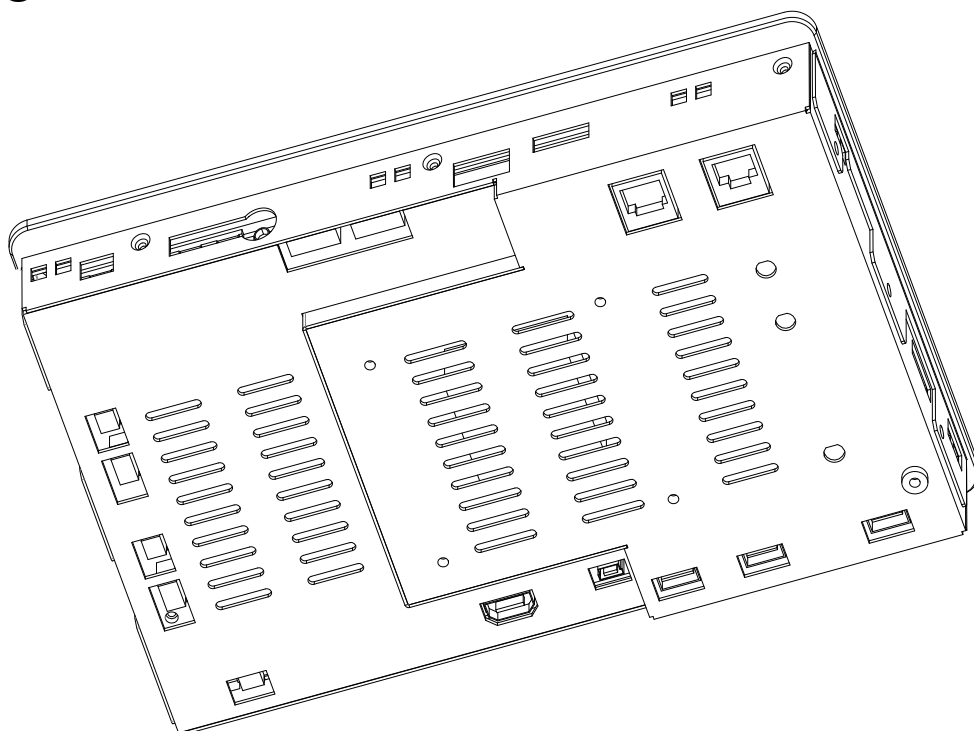
③背面整机示意图
