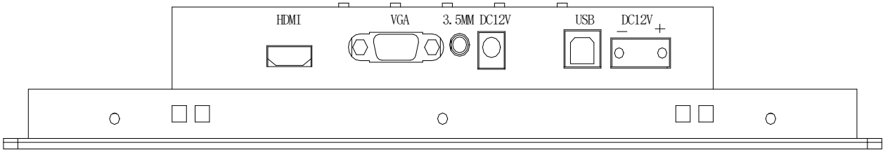
接口示意:
