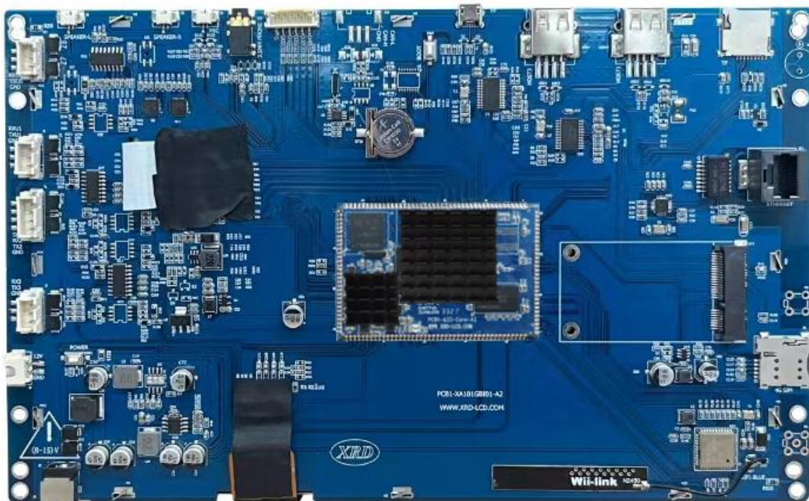
图-2 背面图
