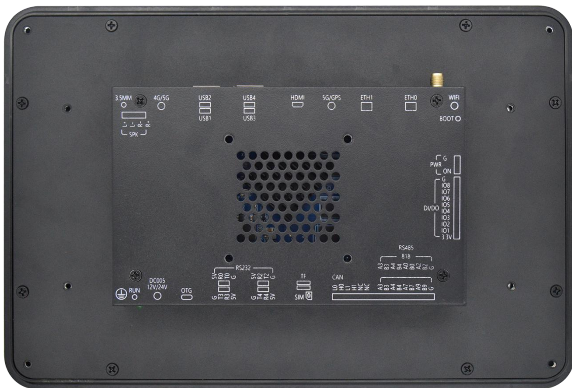
图-2 背面图
