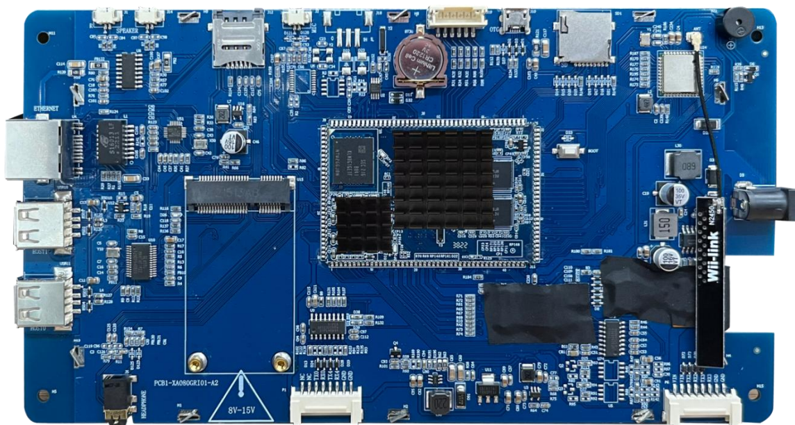
图-2 背面图
