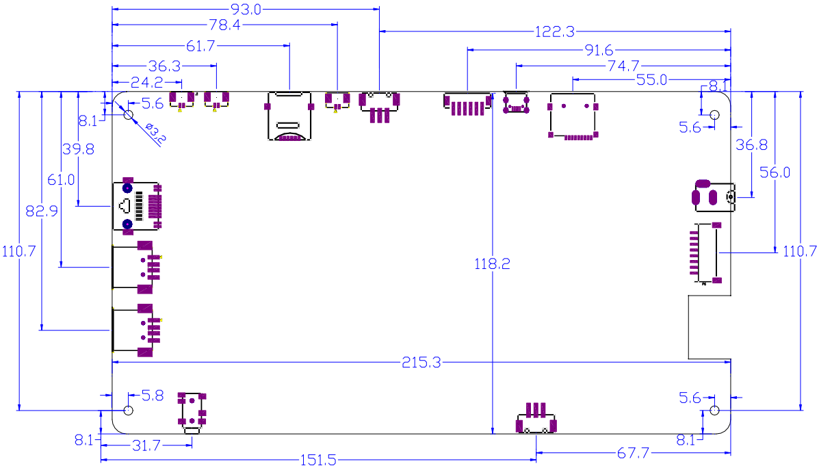
②正视图
